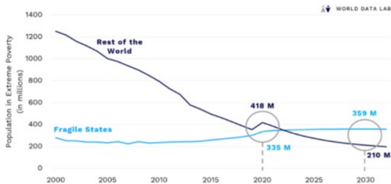
Graphique 2. Evolution de la pauvreté absolue mondiale
